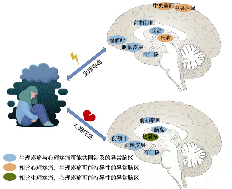
图 1 抑郁症患者生理疼痛和心理疼痛可能涉及的主要异常脑区
